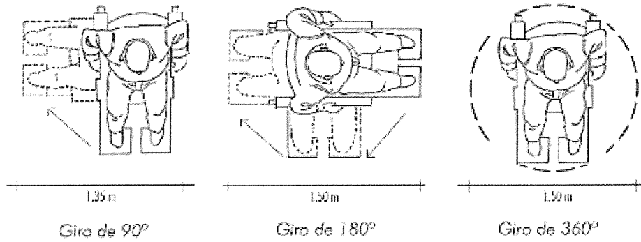
Figura N° 20. Radio de giro de silla de ruedas
