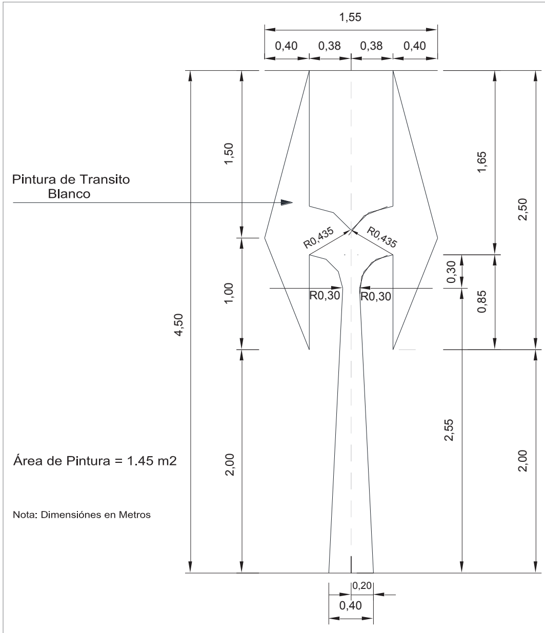
Figura 3.46 Dimensiones de flecha de giro a la derecha e izquierda
