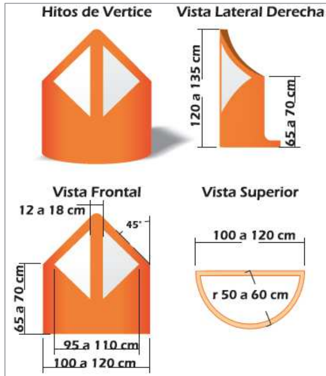
Figura 5.10 Ejemplo de hitos de vértice con dimensiones
