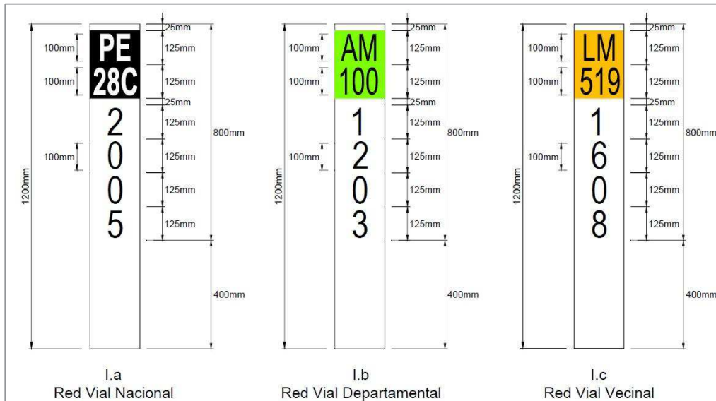
Figura 2.44 Postes de kilometraje (I-2A)
