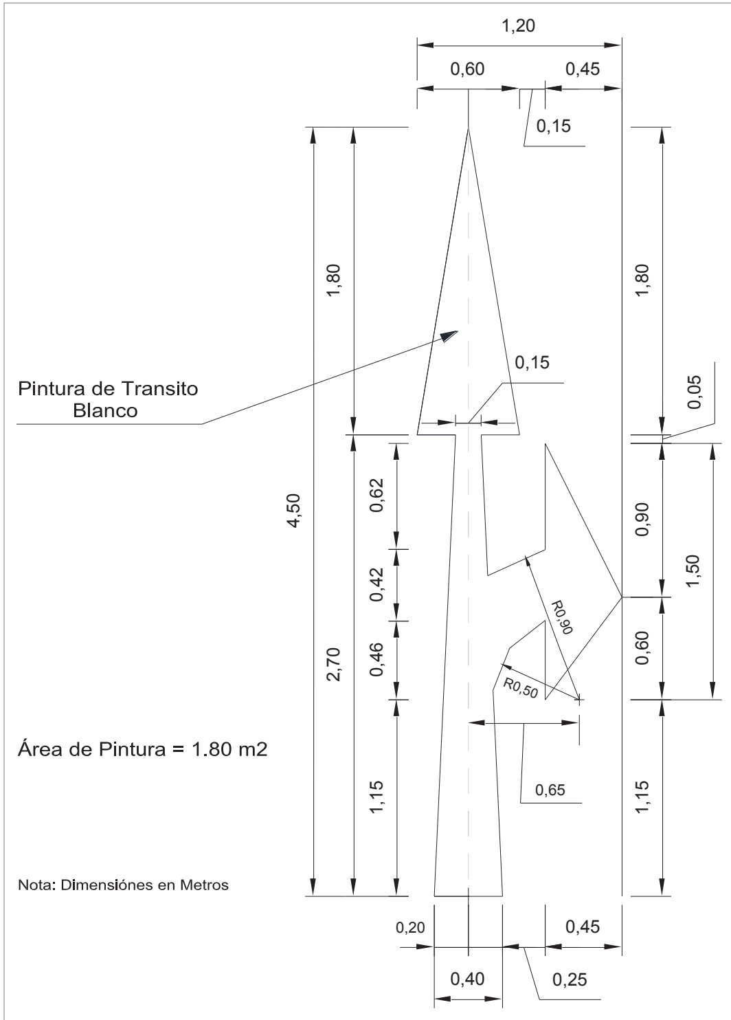
Figura 3.47 Dimensiones de combinación de flecha recta y de giro Flecha recta y de giro (70 km/h o mayor)
