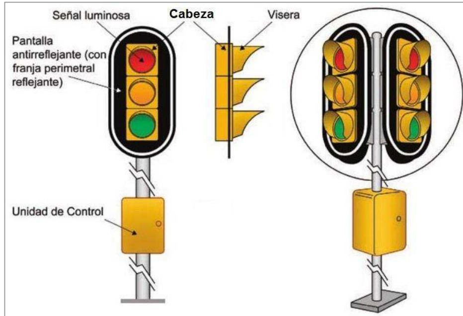
Figura 6.3 Ejemplo de configuración de cabeza de semáforos
