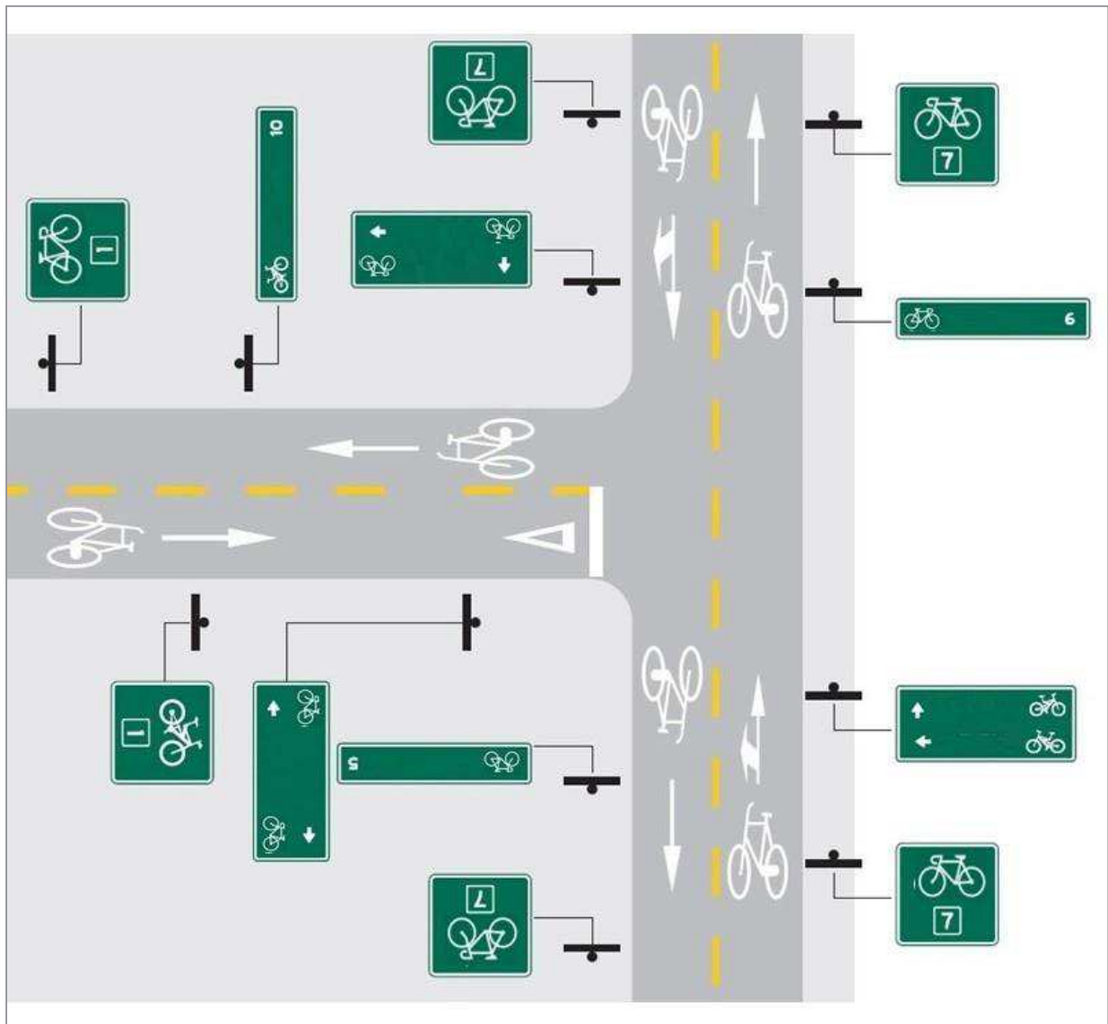
Figura 4.4 Ejemplo de aplicación de una señalización en una intersección de "CICLOVÍAS".
