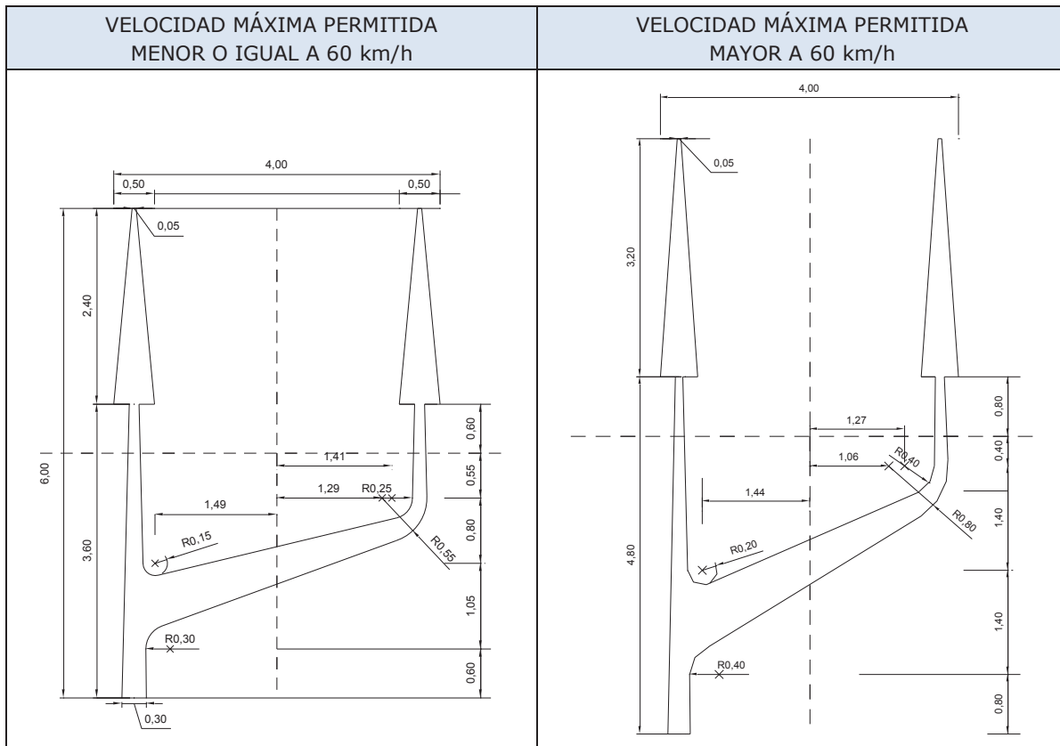
Figura 3.51 Dimensiones de flecha incorporación a carriles exclusivos
