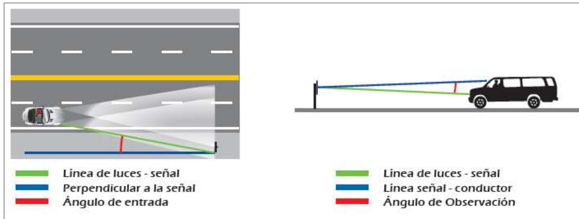
Figura 2.3 Retrorreflexión
