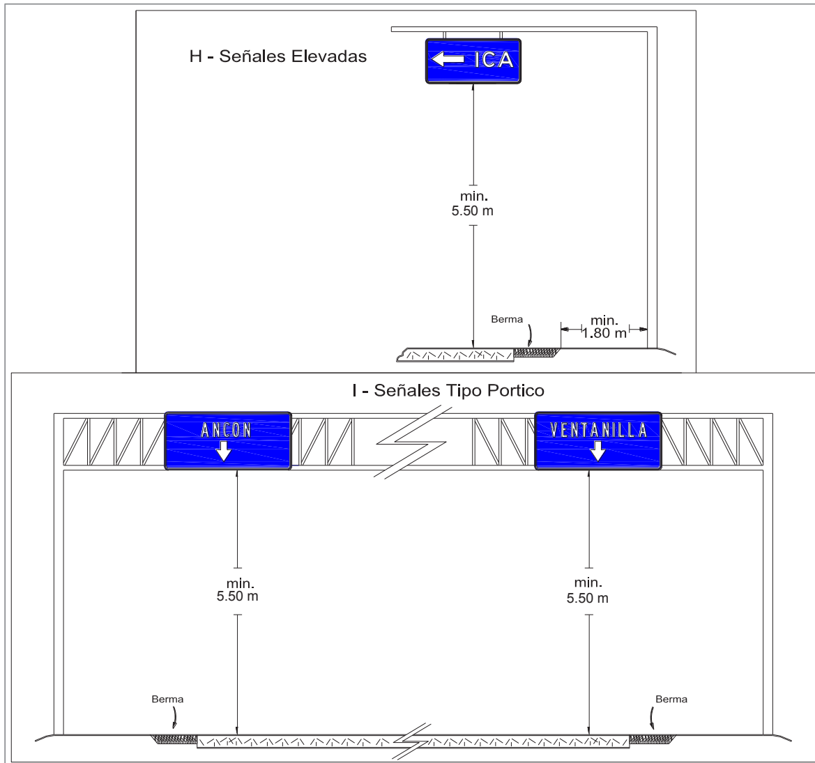
(Continua) Figura 2.5 Ejemplo de Ubicación Lateral
