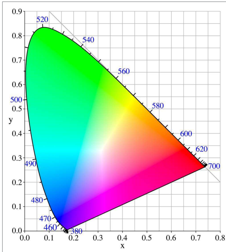
Figura 2.2 Diagrama Cromático CIE 1931
