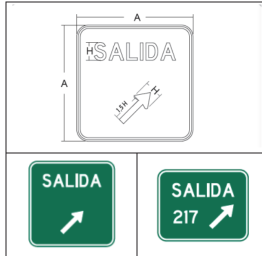
Figura 2.37 Ejemplo de señales salida inmediata
