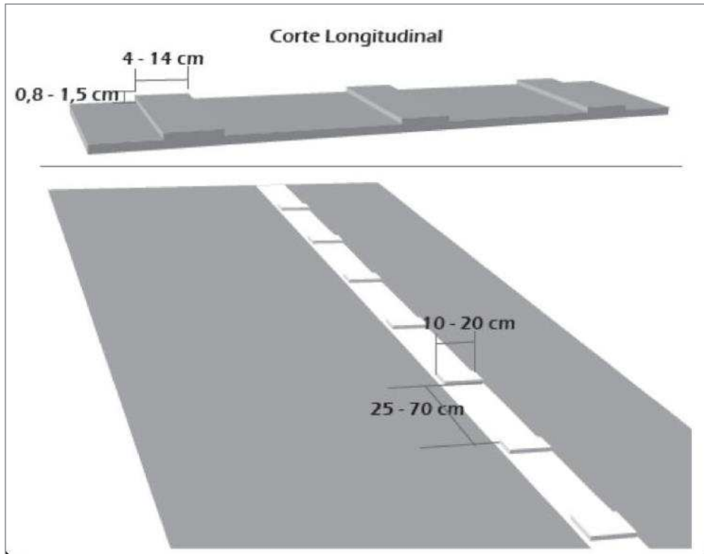
Figura 3.57 Ejemplo de demarcación bajo relieve
